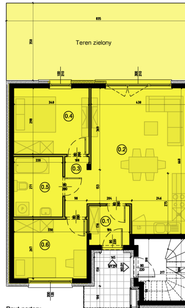
Rzut parteru
