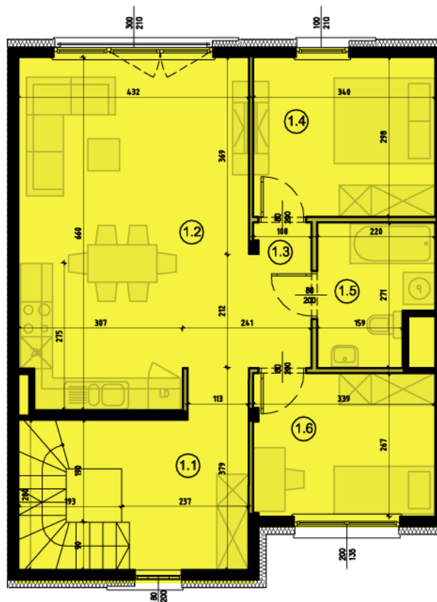
Rzut piętra
