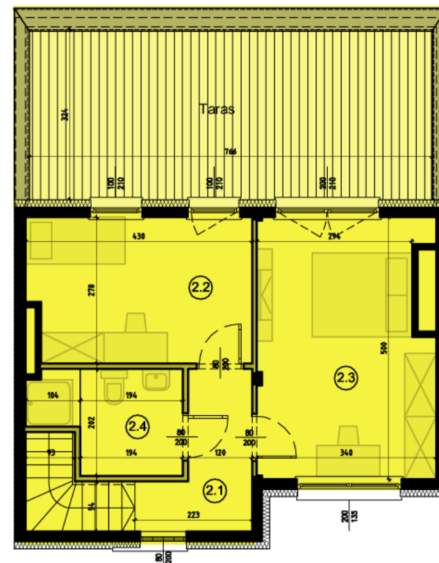
Rzut poddasza
