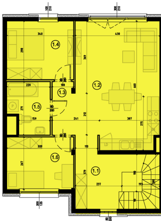
Rzut piętra
