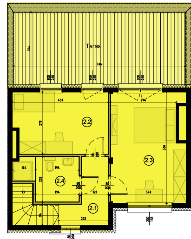
Rzut poddasza
